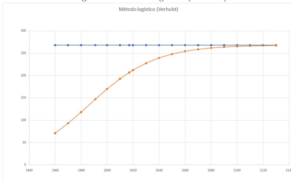
Figura 4.3: Modelo logístico (Verhulst)
