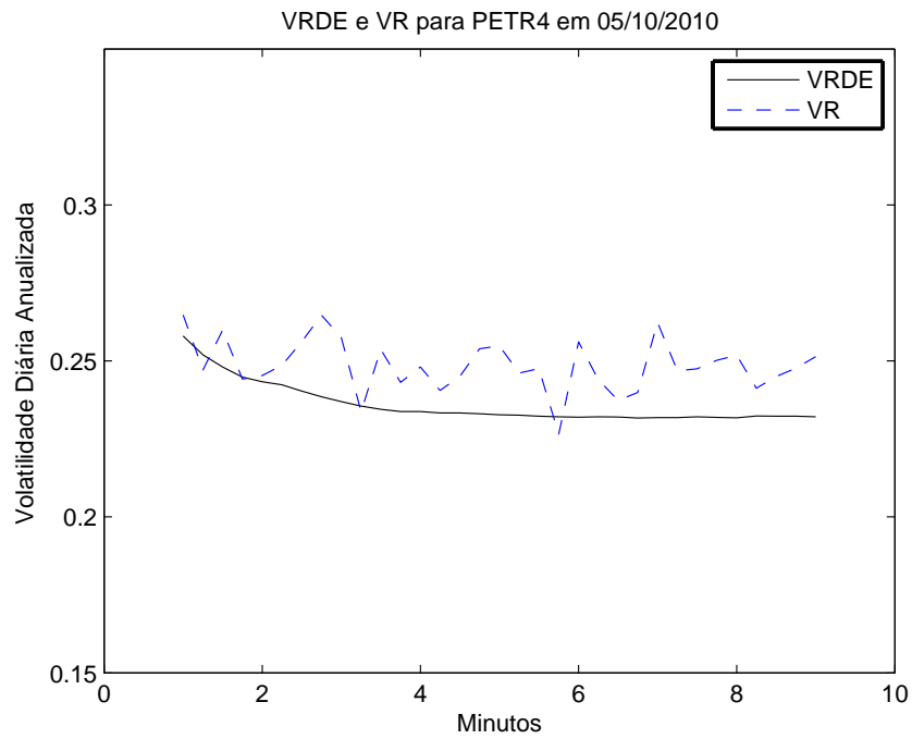
Figura 4.7: Estimação da VRDE e VR para PETR4 em 05/10/2010.
