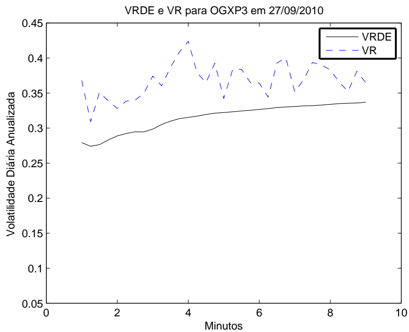
Figura 4.23: Estimação da VRDE e VR para OGXP3 em 27/09/2010.
