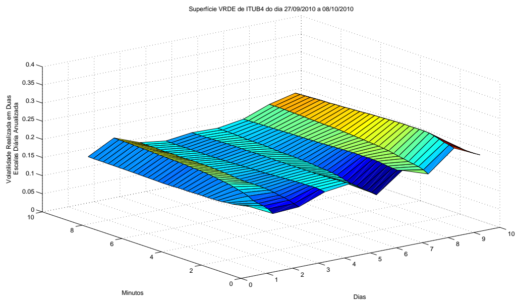
Figura 4.44: Superfície de VRDE dos 10 dias de transação e por intervalo de tempo utilizado na estimação.
