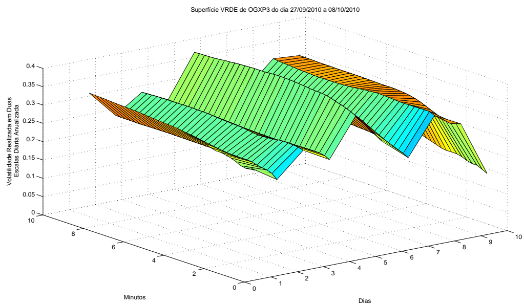
Figura 4.33: Superfície de VRDE dos 10 dias de transação e por intervalo de tempo utilizado na estimação.
