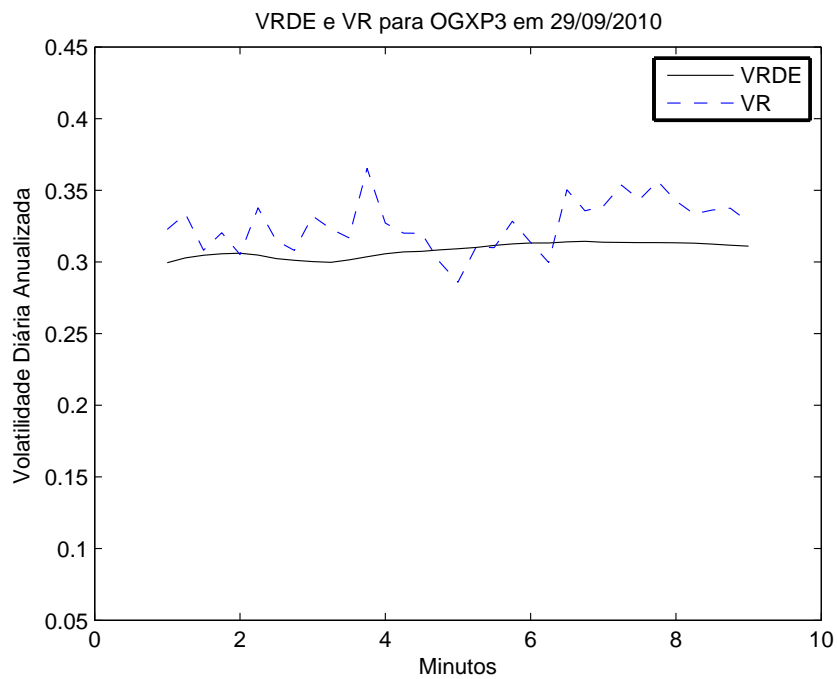
Figura 4.25: Estimação da VRDE e VR para OGXP3 em 29/09/2010.
