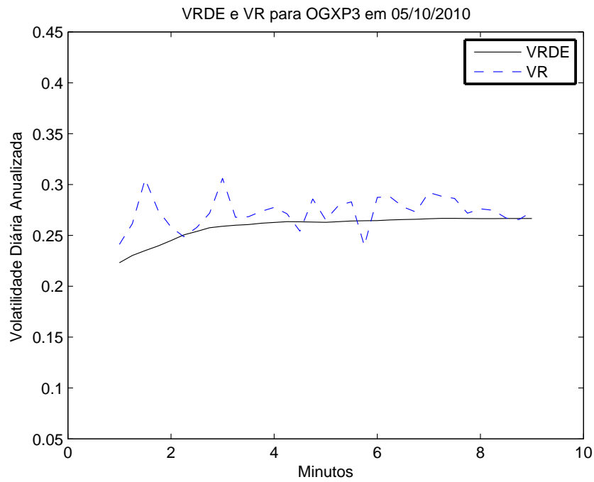
Figura 4.29: Estimação da VRDE e VR para OGXP3 em 05/10/2010.
