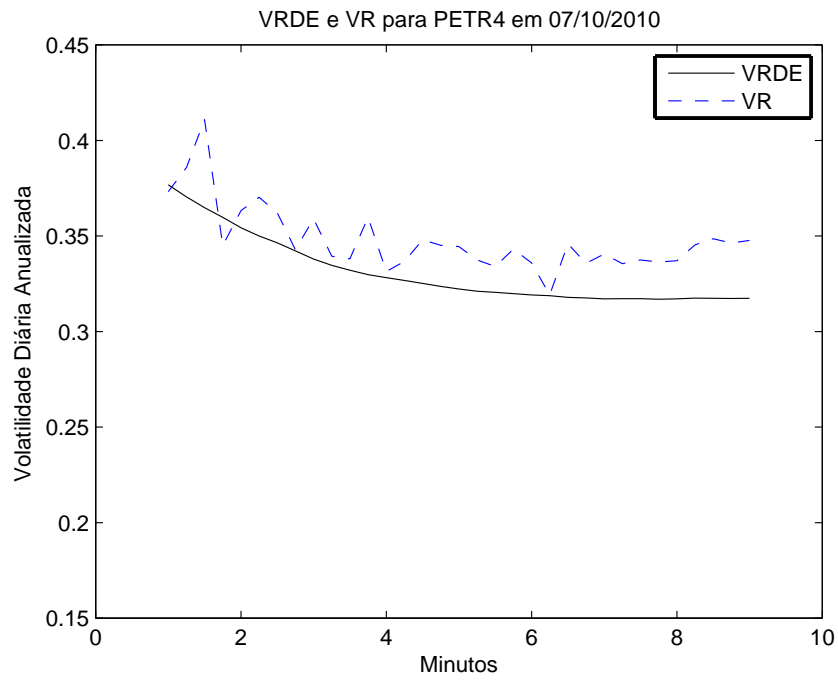
Figura 4.9: Estimação da VRDE e VR para PETR4 em 07/10/2010.
