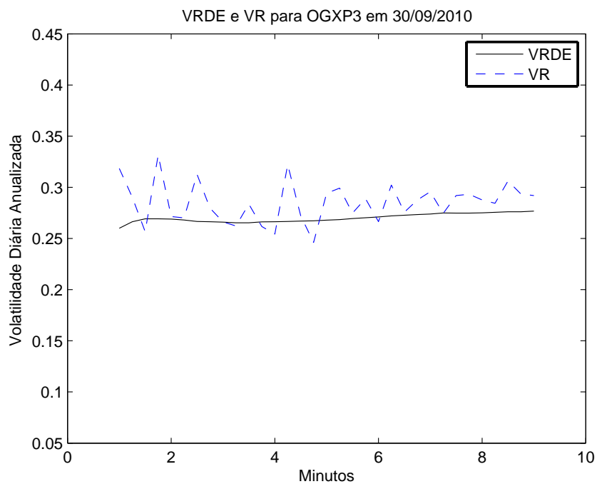
Figura 4.26: Estimação da VRDE e VR para OGXP3 em 30/09/2010.
