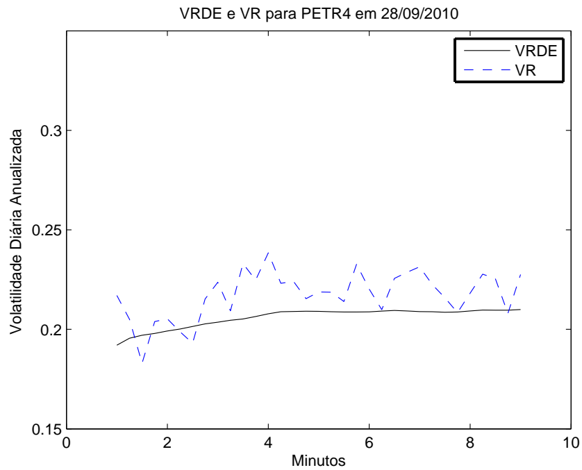
Figura 4.2: Estimação da VRDE e VR para PETR4 em 28/09/2010.
