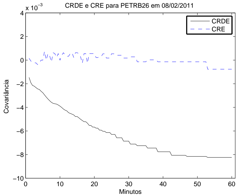
Figura 5.3: Estimação da CRDE (Eq. (5.28)-(5.30)) e CRE (Eq. (5.31)) para PETRB26 em 08/02/2011.
