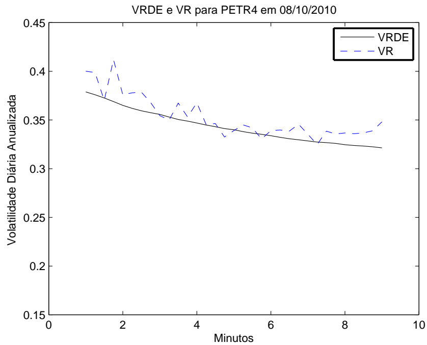
Figura 4.10: Estimação da VRDE e VR para PETR4 em 08/10/2010.
