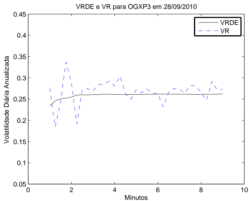
Figura 4.24: Estimação da VRDE e VR para OGXP3 em 28/09/2010.
