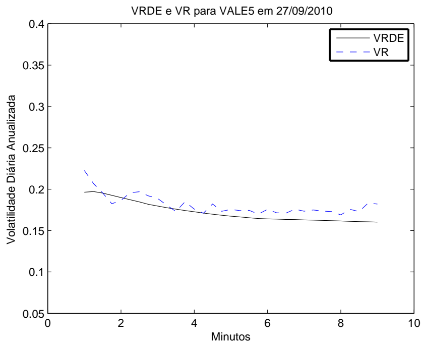
Figura 4.12: Estimação da VRDE e VR para VALE5 em 27/09/2010.
