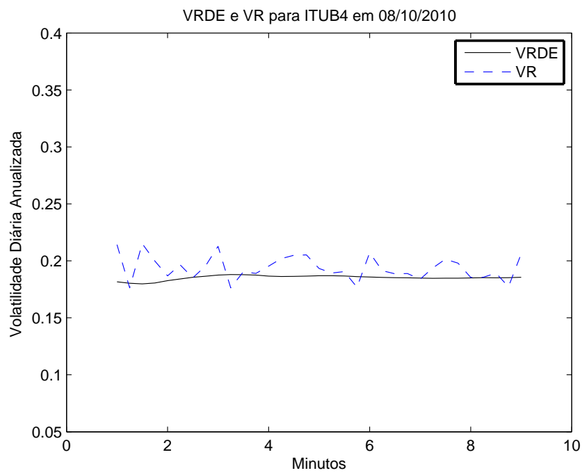
Figura 4.43: Estimação da VRDE e VR para ITUB4 em 08/10/2010.
