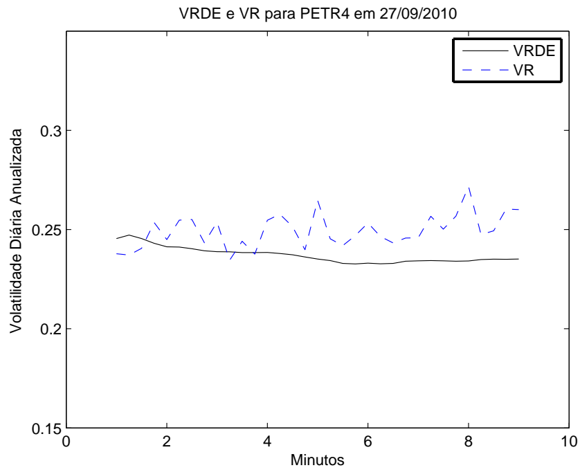
Figura 4.1: Estimação da VRDE e VR para PETR4 em 27/09/2010.
