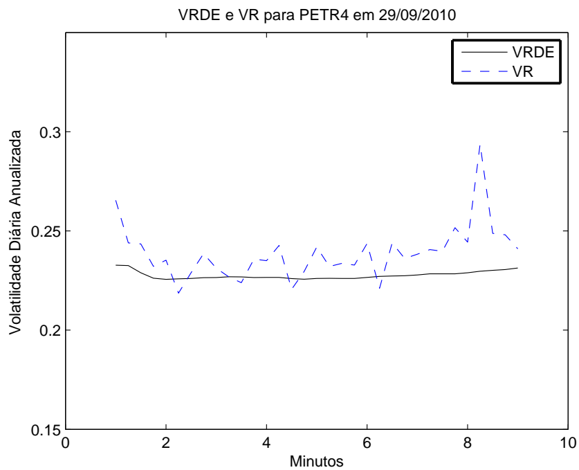
Figura 4.3: Estimação da VRDE e VR para PETR4 em 29/09/2010.
