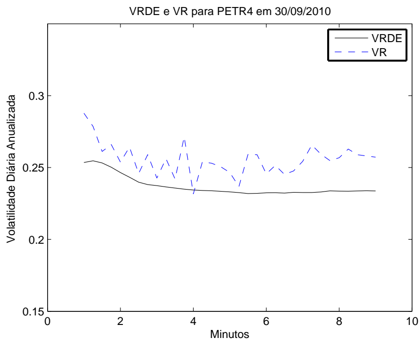
Figura 4.4: Estimação da VRDE e VR para PETR4 em 30/09/2010.
