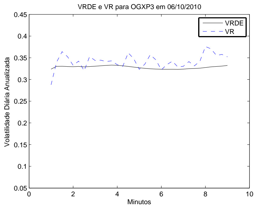
Figura 4.30: Estimação da VRDE e VR para OGXP3 em 06/10/2010.
