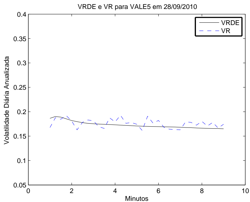
Figura 4.13: Estimação da VRDE e VR para VALE5 em 28/09/2010.
