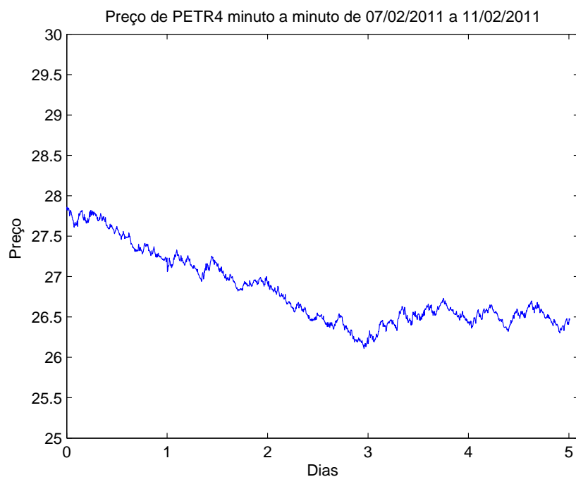
Figura 5.1: Preço de PETR4, minuto a minuto de 07/02/2011 a 11/02/2011
