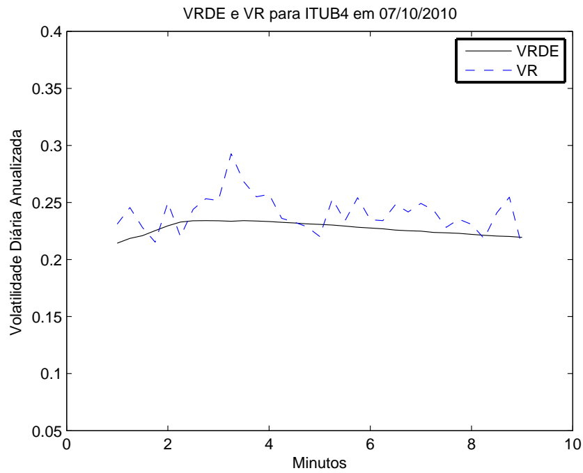
Figura 4.42: Estimação da VRDE e VR para ITUB4 em 07/10/2010.
