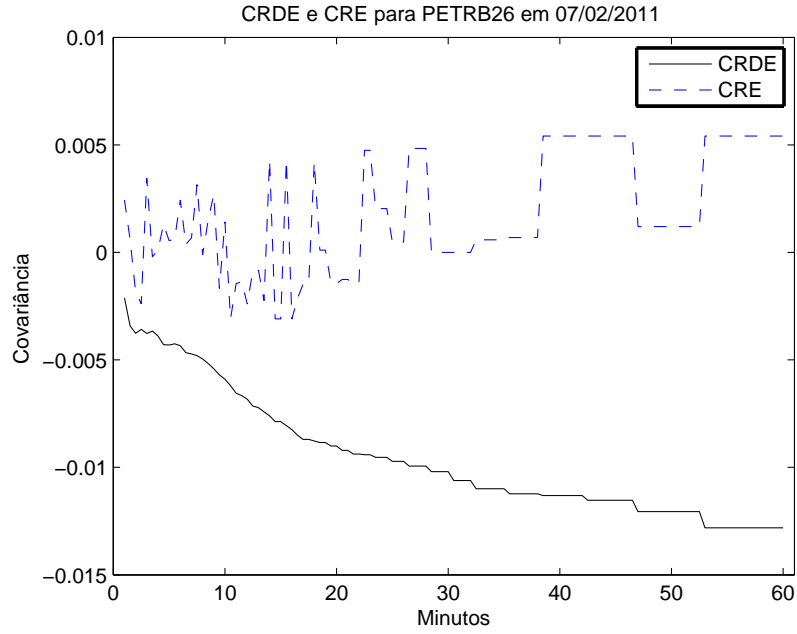
Figura 5.2: Estimação da CRDE (Eq. (5.28)-(5.30)) e CRE (Eq. (5.31)) para PETRB26 em 07/02/2011.
