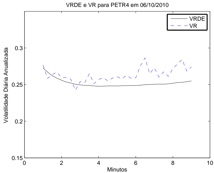
Figura 4.8: Estimação da VRDE e VR para PETR4 em 06/10/2010.
