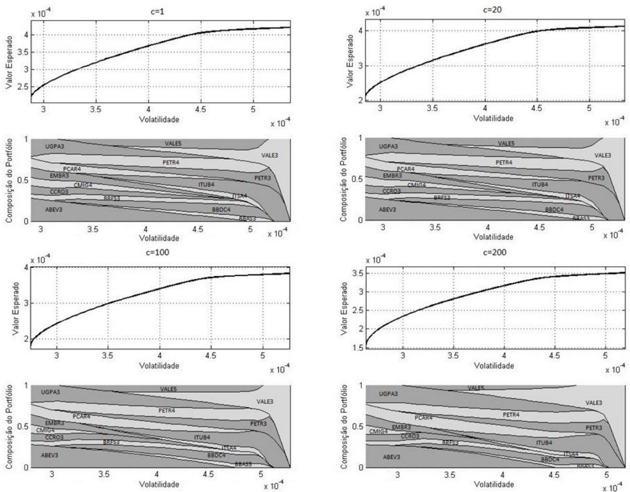
Figura 4.3: Fronteira Eficiente: Modelo de Black-Litterman sem Incorporação das Visões.
