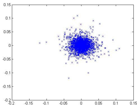
Figura 5.16: Gráfico de Dispersão ABEV3
