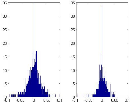
Figura 5.13: Séries do Ativo UGPA3
