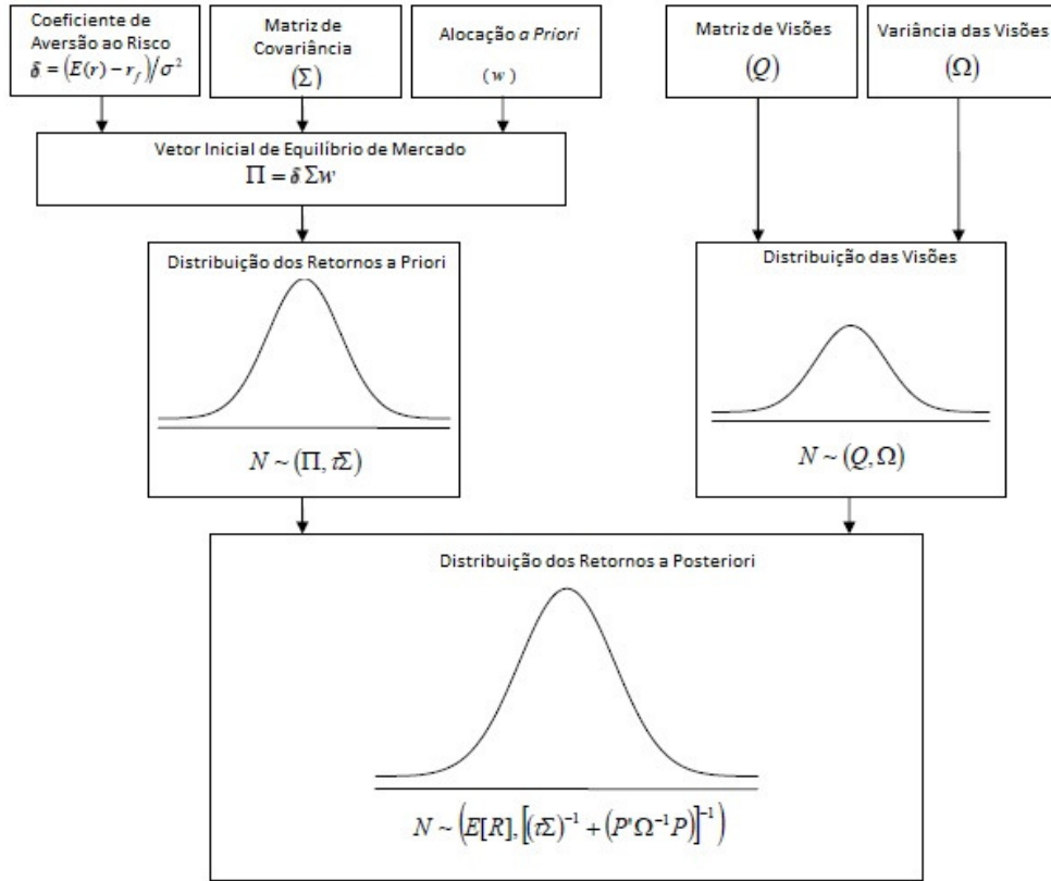
Figura 2.4: Derivação dos Retornos a posteriori : Modelo de Black-Litterman
