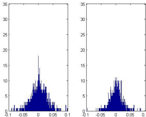
Figura 5.15: Séries do Ativo VALE5
