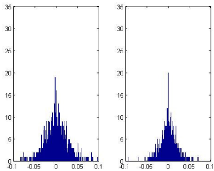
Figura 5.3: Séries do Ativo BBDC4
