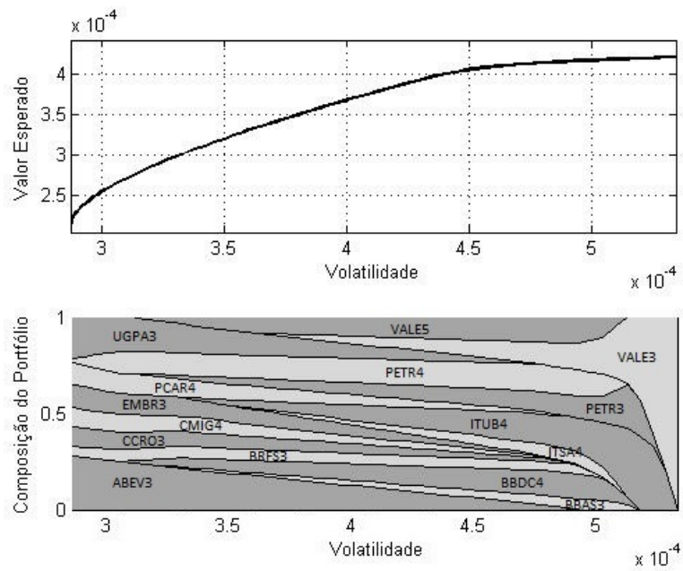
Figura 4.3: Fronteira Eficiente: Modelo de Black-Litterman sem Incorporação das Visões.
