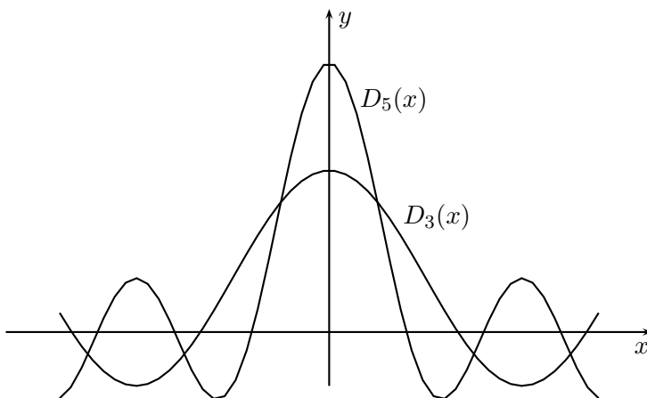
Figura 2.2: Núcleos de Dirichlet
