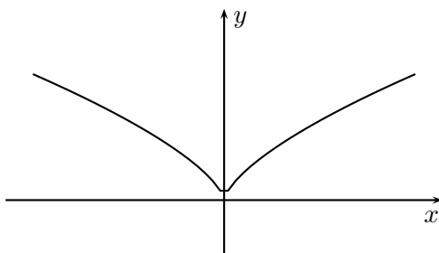
Figura 4.2: Curva não regular
