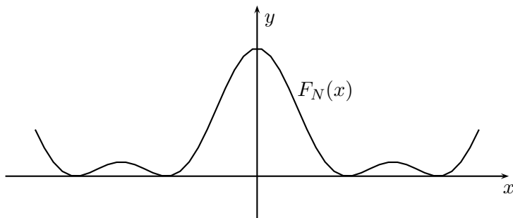
Figura 2.3: Núcleo de Fejér
