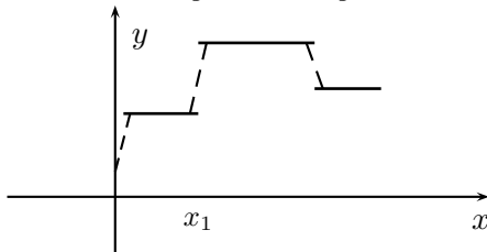
Figura 1.3: Construção de uma aproximação contínua
