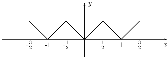
Figura 2.1: Gráfico da função f(x) = |x| , f(x) = f(x + 1) .
